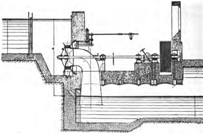
Fig. 48. Francis-Turbine mit liegender Welle der Maschinenfabrik Augsburg.
